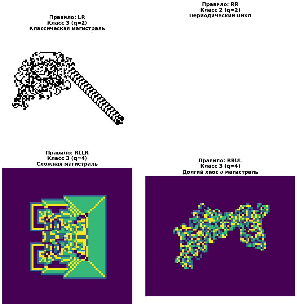
Рис. 1: Галерея режимов: классическая магистраль LR ( q = 2 ); пустое поле правила RR на шаге 200 = 25\tau (визуальное доказательство периодичности: поле вернулось в начальное состояние); структурированный фронт RLLR ( q = 4 ); долгий хаос правила RRUL ( q = 4 ).
